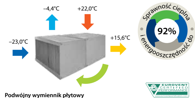
Podwójny wymiennik płytowy
